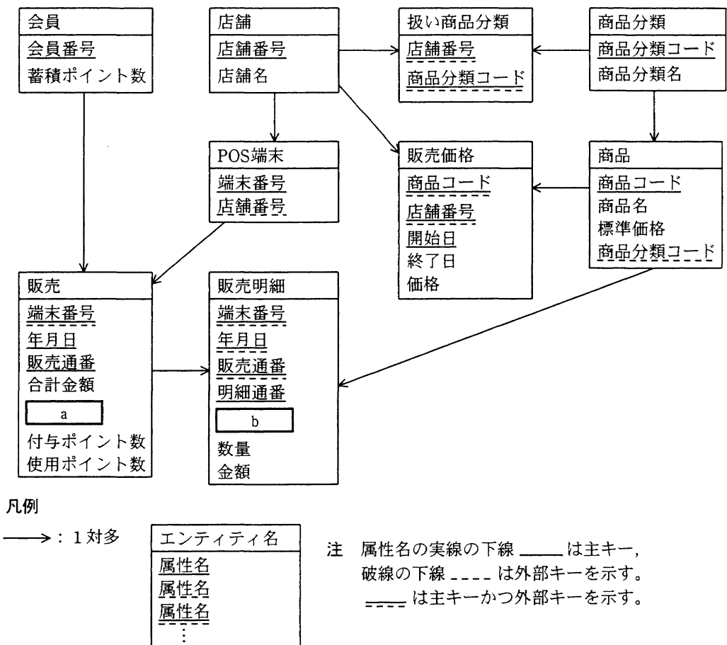
図 本システムのE-R図
