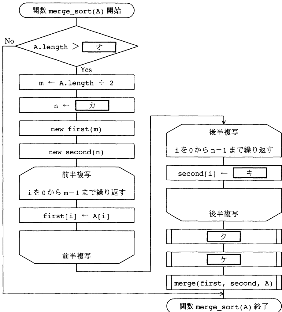
図4 関数 merge_sort のアルゴリズム
