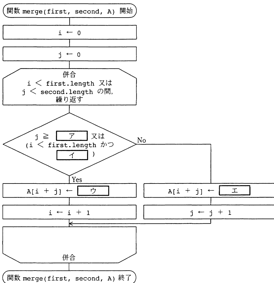
図 3 関数 merge のアルゴリズム
