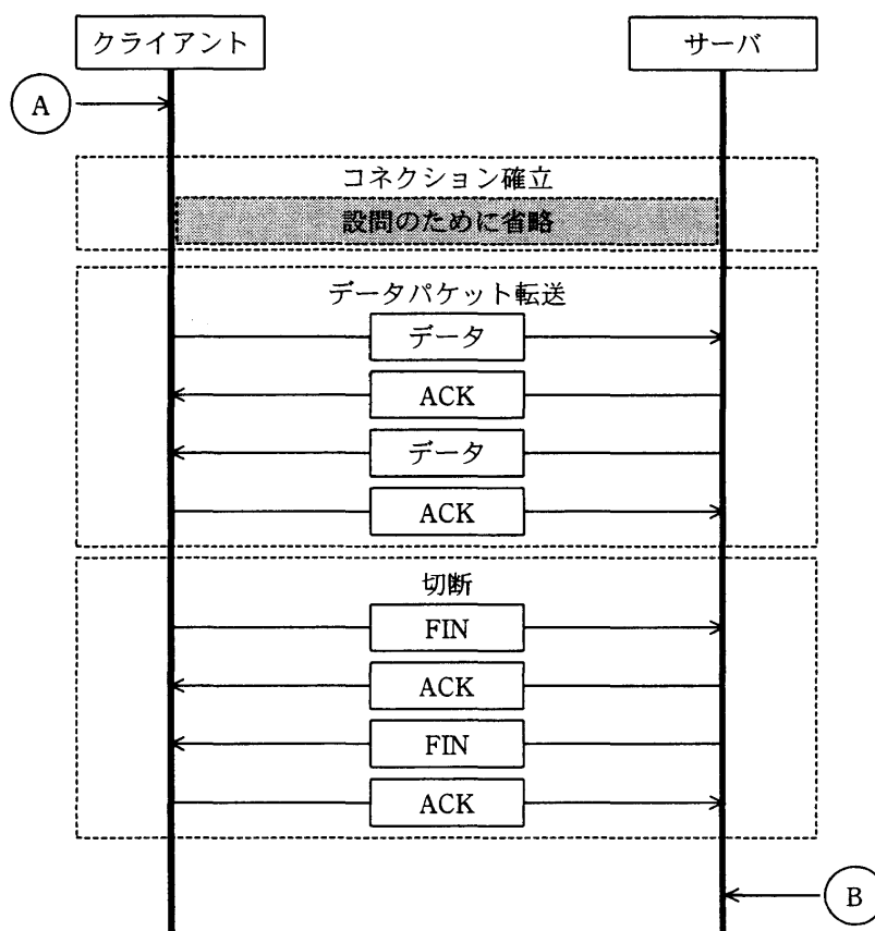
図2 TCP パケットシーケンス
