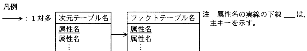
図 2 データウェアハウスのスタースキーマ
