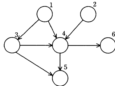
図 5 有向グラフ2
