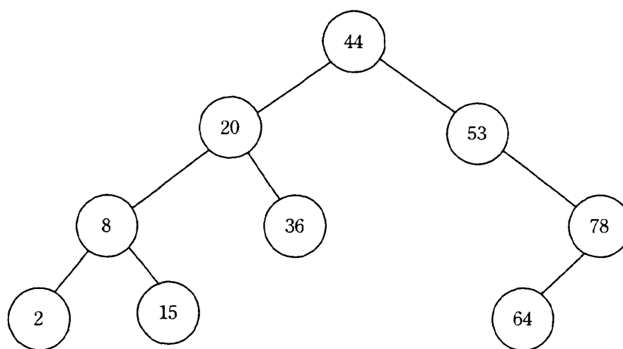
図1 2分探索木の例
