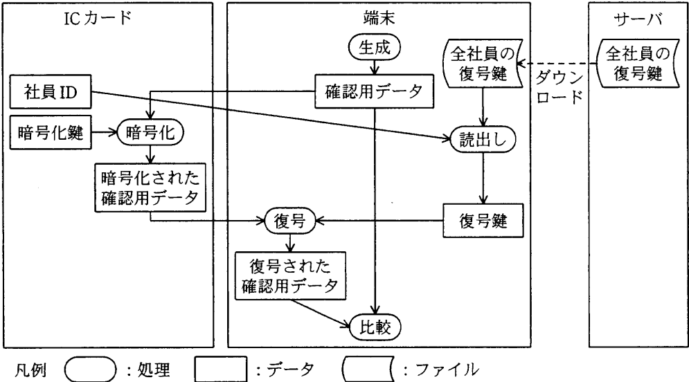
図 ICカードの認証方式
