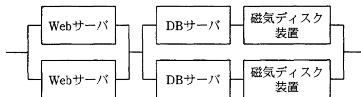
図 3 検討案 1 の信頼性モデル
