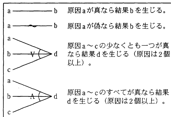
図 2 原因結果グラフで使う記号
