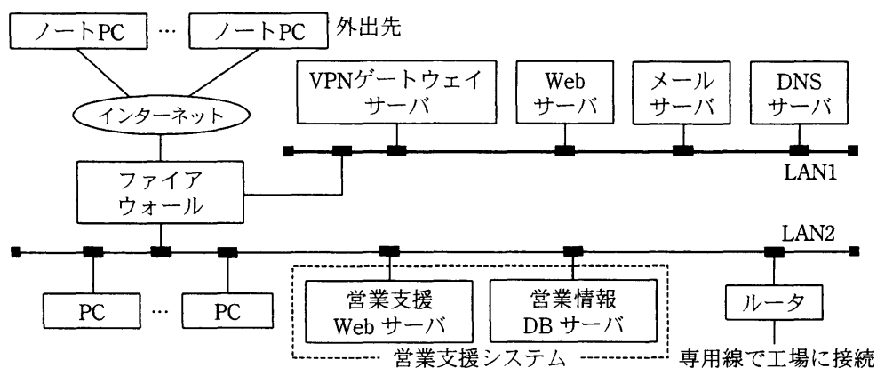
図1 W社本社ビルの情報システムの構成
