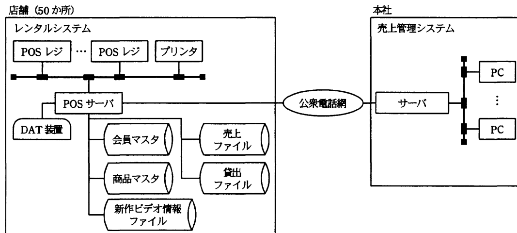
図1 G社のシステム構成
