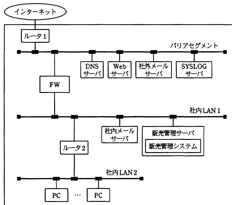
図 W社のシステム構成
