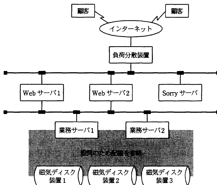
図2 強化後の注文システム構成
