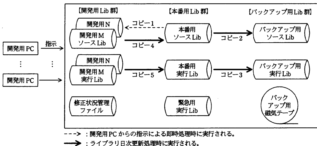
図 変更後のライブラリ管理システムの概要
