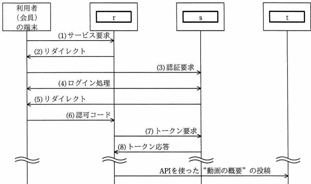
図 10 OAuth2 を用いた T 社投稿サイトと X 社動画サーバの連携の流れ
