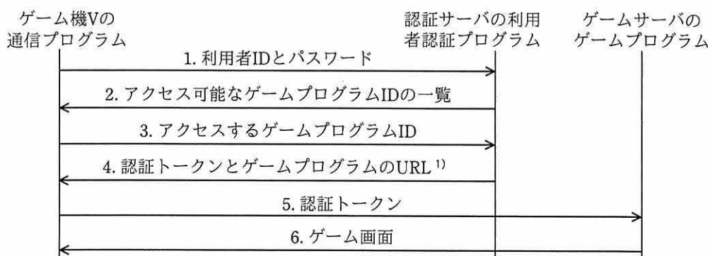
図 2 利用者がゲームを行う際の認証フロー
