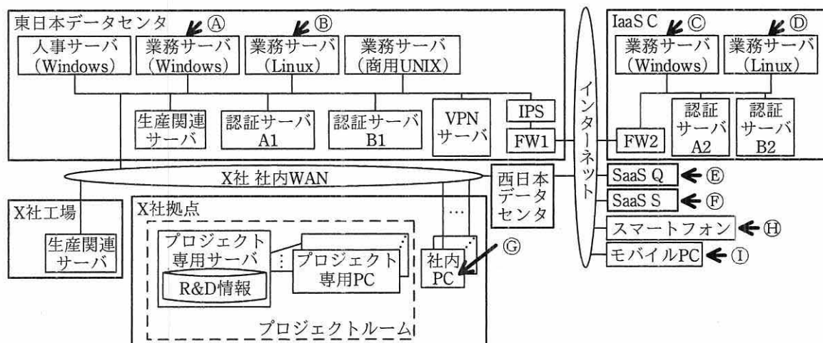
図 3 モバイル環境を含む日本国内のハイブリッドクラウド環境の論理構成
