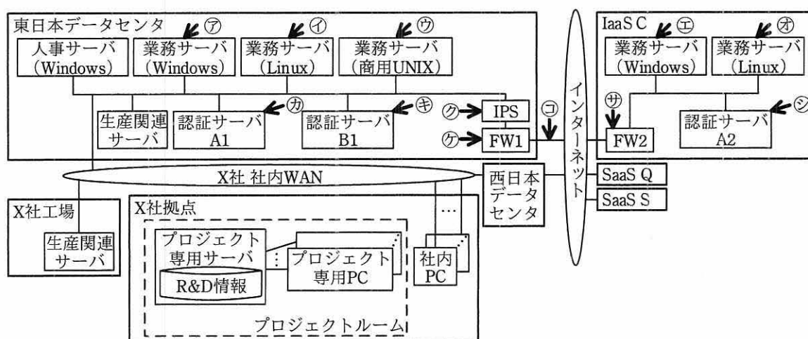
図 2 案 1 における日本国内のハイブリッドクラウド環境の論理構成
