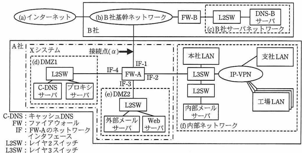
図1 A社及びB社サービスのネットワーク構成
