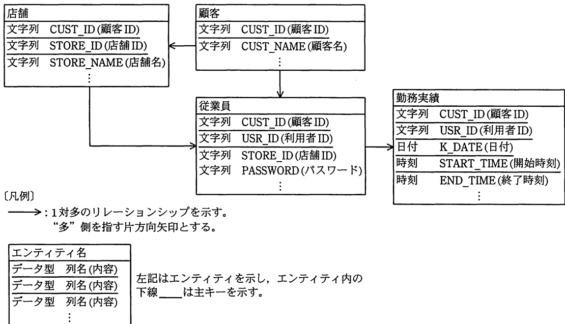
図 6 主なテーブルの E-R 図
