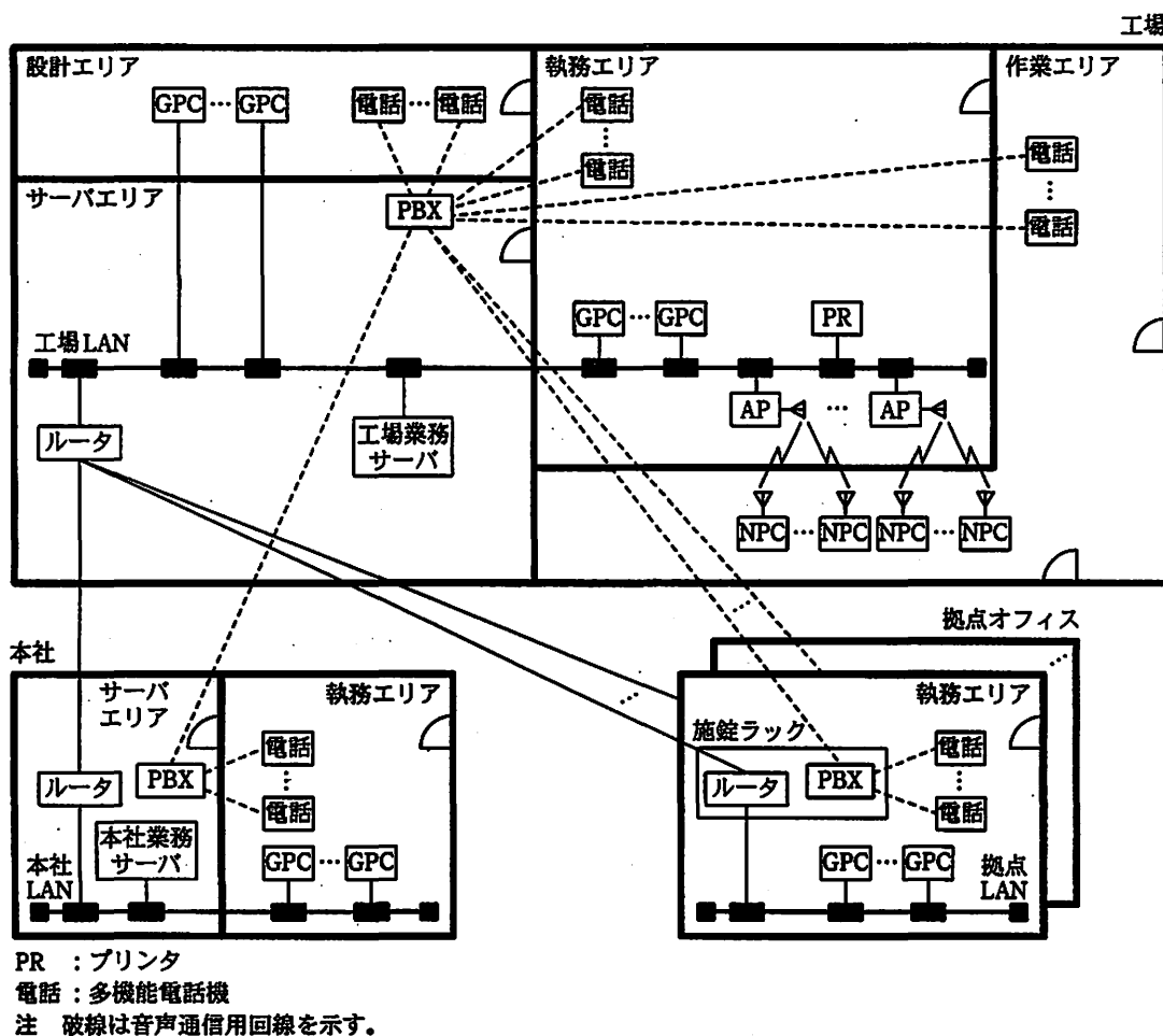
図1 S ネットワークと内線電話の構成
