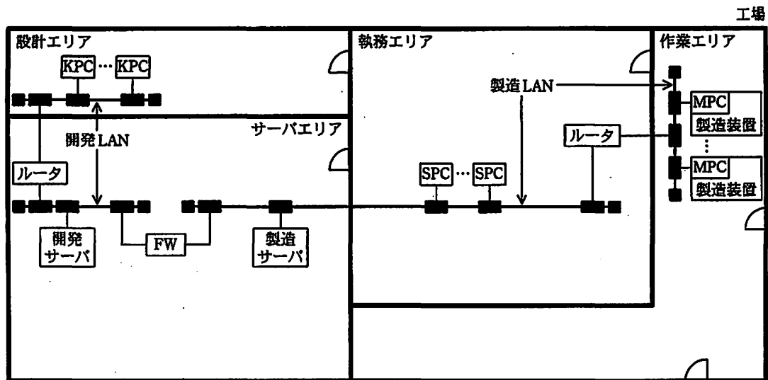
図2 Tネットワークの構成
