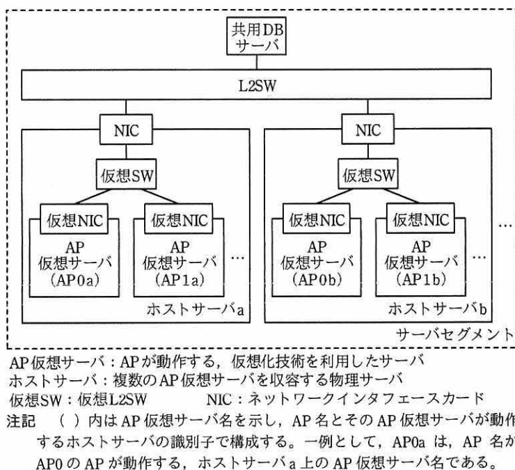
図 2 サーバ仮想化技術を利用した AP の構成
