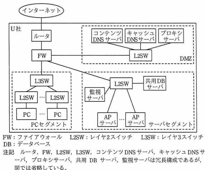
図1 現在のU社ネットワーク構成（抜粋）
