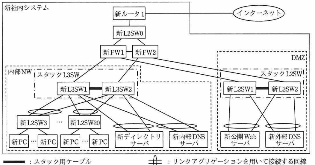
図 3 新社内システムの構成（抜粋）
