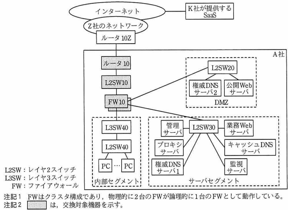
図1 現在の A 社ネットワーク環境（抜粋）
