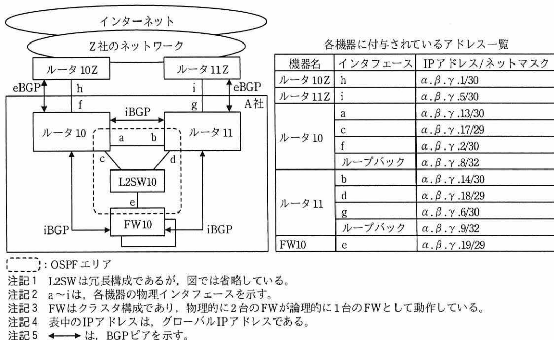
図2 Z社の提案した構成（抜粋）
