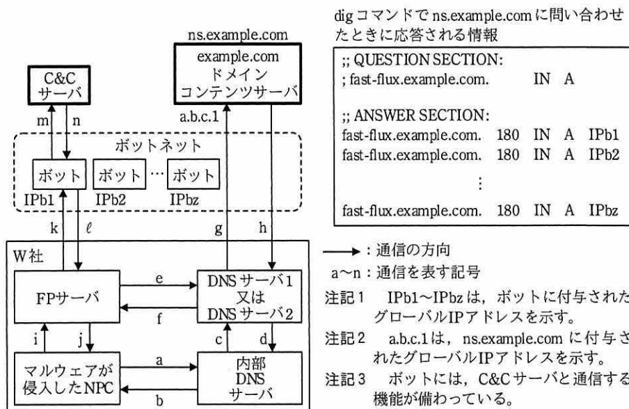
図 4 Fast Flux 手法が用いられたときのマルウェアによる C&C サーバとの通信例 (抜粋)
