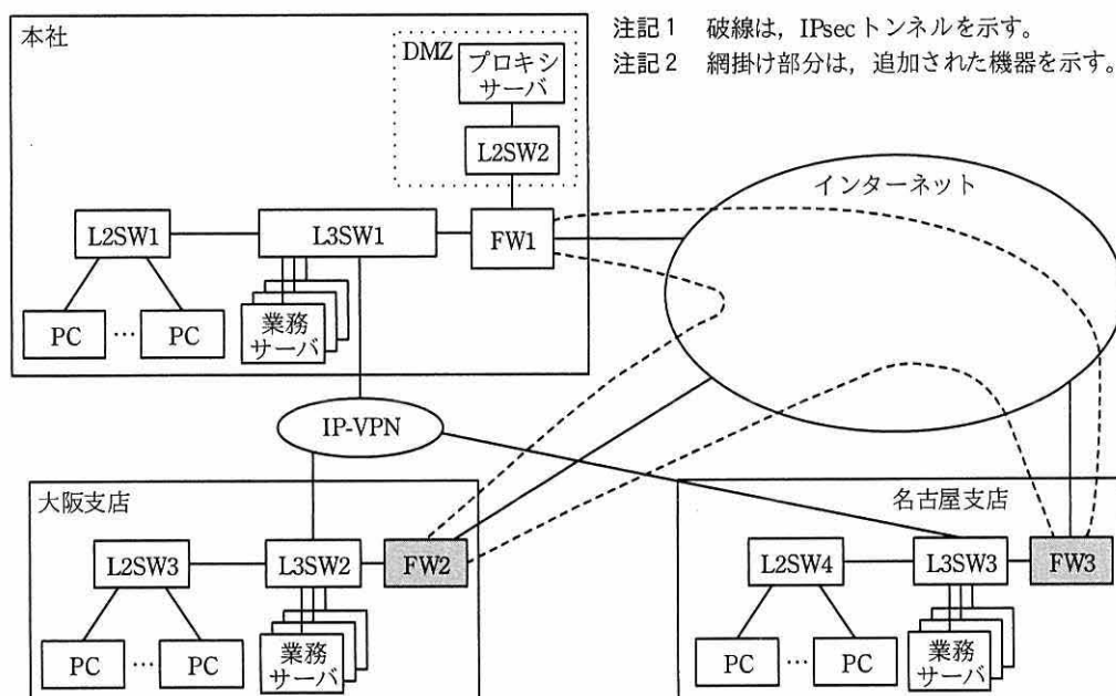
図2 Eさんが考えたD社のネットワーク構成（抜粋）
