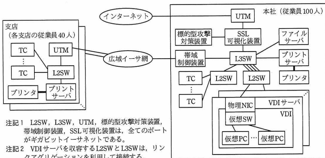
図2 VDI 導入後のネットワーク構成案（抜粋）
