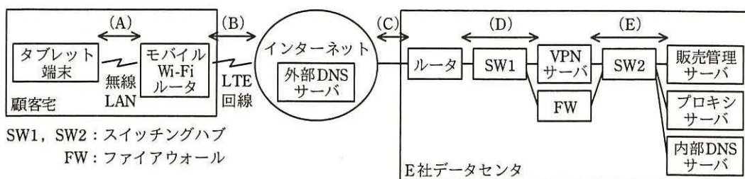
図 1 モバイルネットワーク構成案
