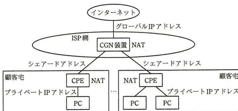
図 2 NAT444 の構成
