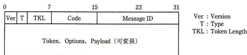
図 7 CoAP のメッセージ形式
