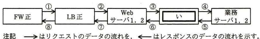
図3 通常時のサーバへのアクセスに関するデータの流れ
