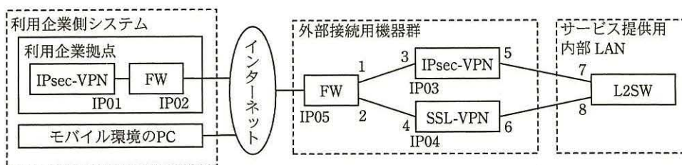
図 6 外部接続用機器の構成図
