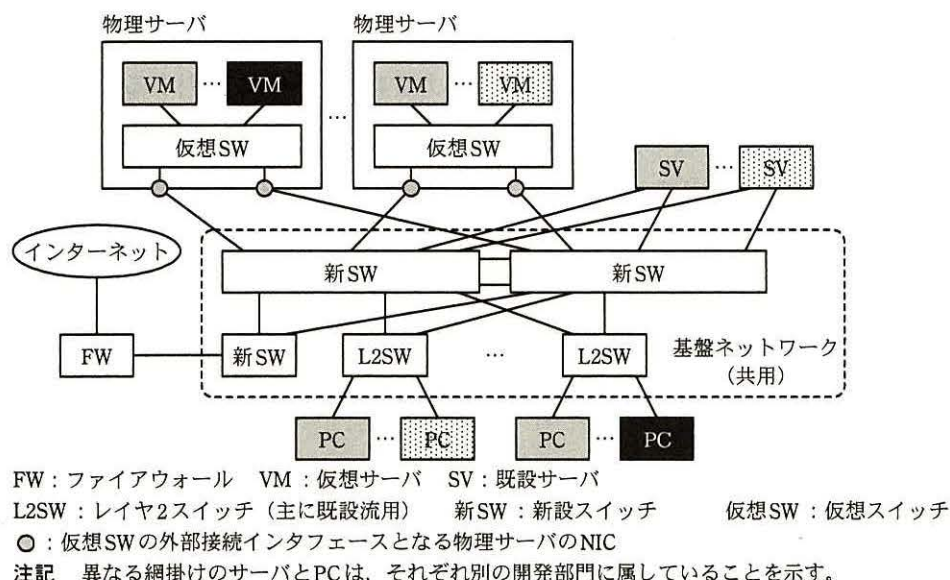
図1 移行後の開発システムの構成（概要）
