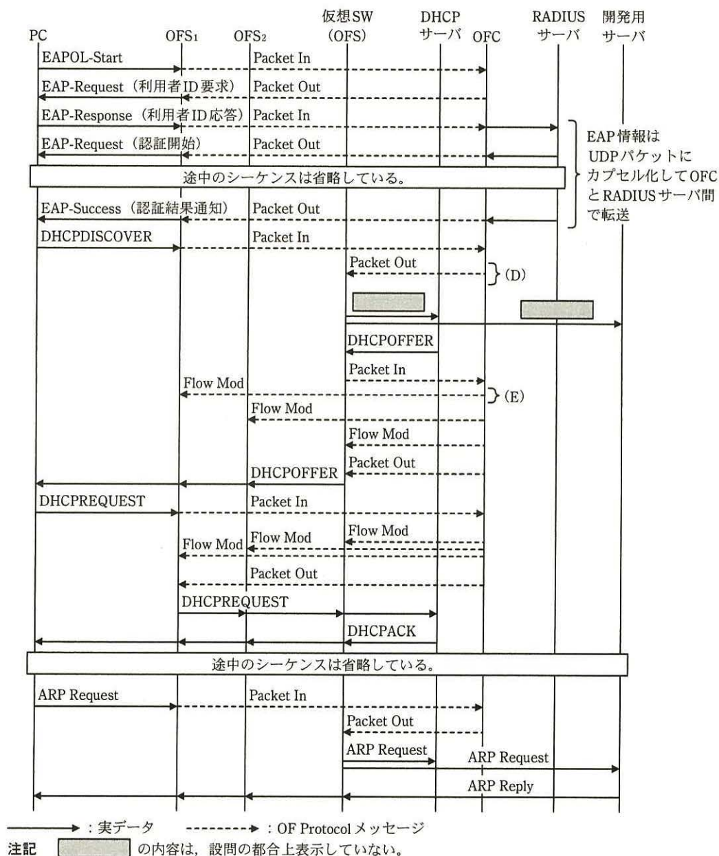
図 6 IEEE 802.1X 認証方式による PC のテナントネットワークへの接続シーケンス例 (概要)
