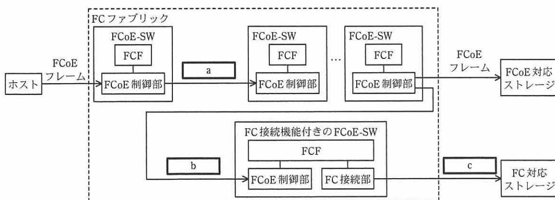
図 5 FCoE-SW による FCoE フレーム及び FC フレームの転送
