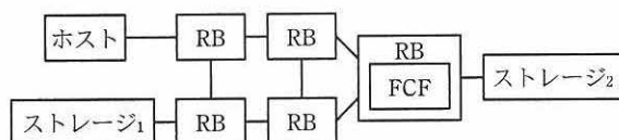
案1 FCF機能付きRBを1か所だけに配置した構成
