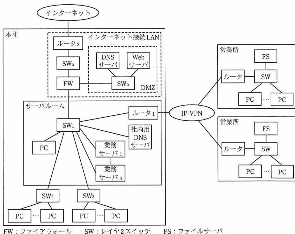
図1 A社の現在のネットワークシステム構成（抜粋）
