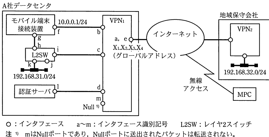
図 4 地域保守会社及び MPC から A 社データセンタへの接続（抜粋）
