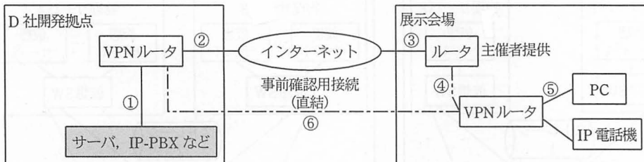
図 4 D 社開発拠点と展示会場間のネットワーク接続構成
