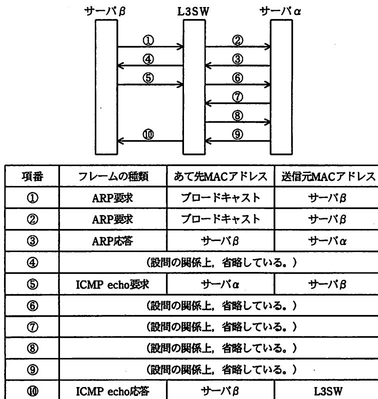
図5 メッセージフロー
