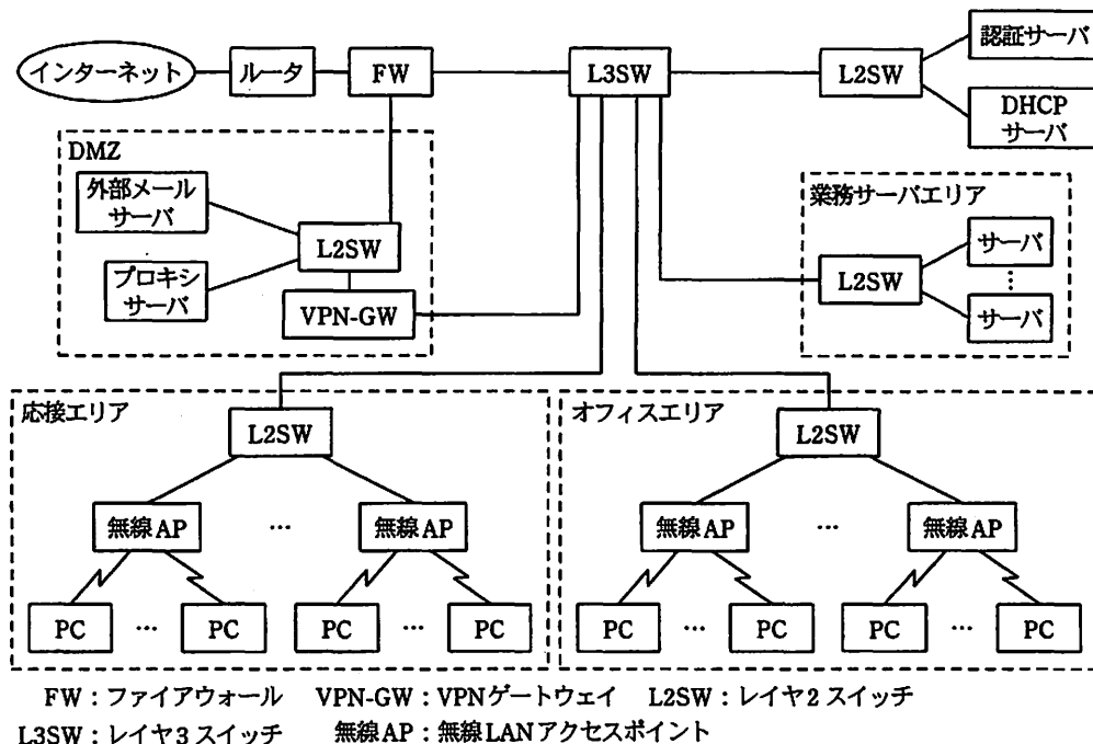
図1 集約後の無線 LAN システム構成図
