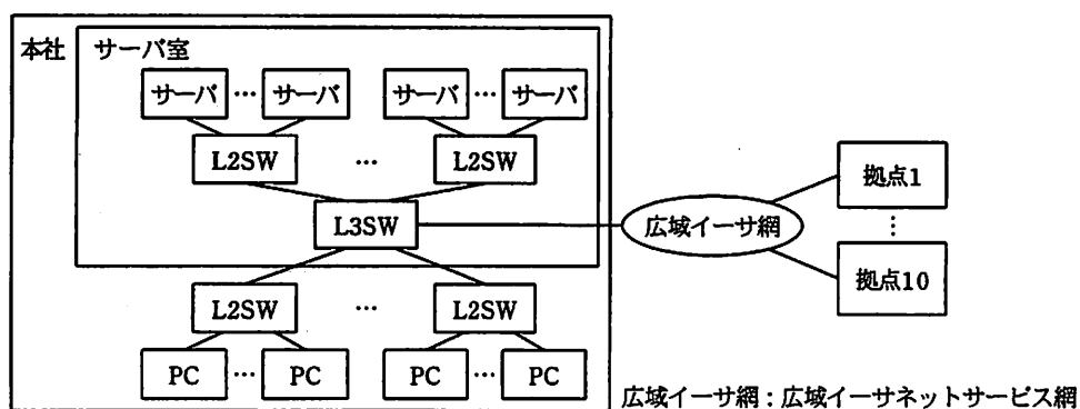
図1 D社ネットワークシステムの概要
