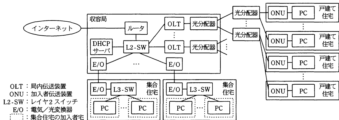
図 X社に提案する光ファイバ網の構成（抜粋）
