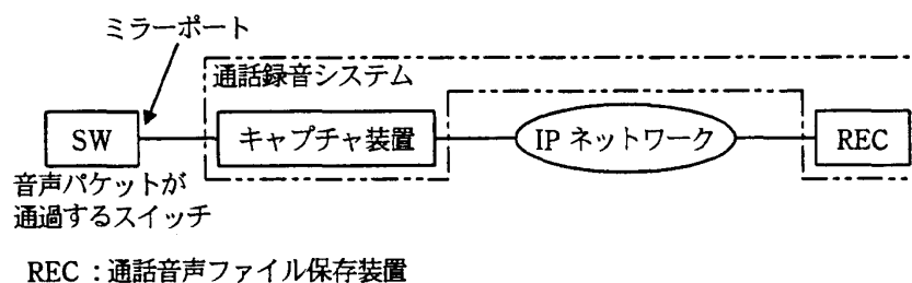
図 2 通話録音システムの構成
