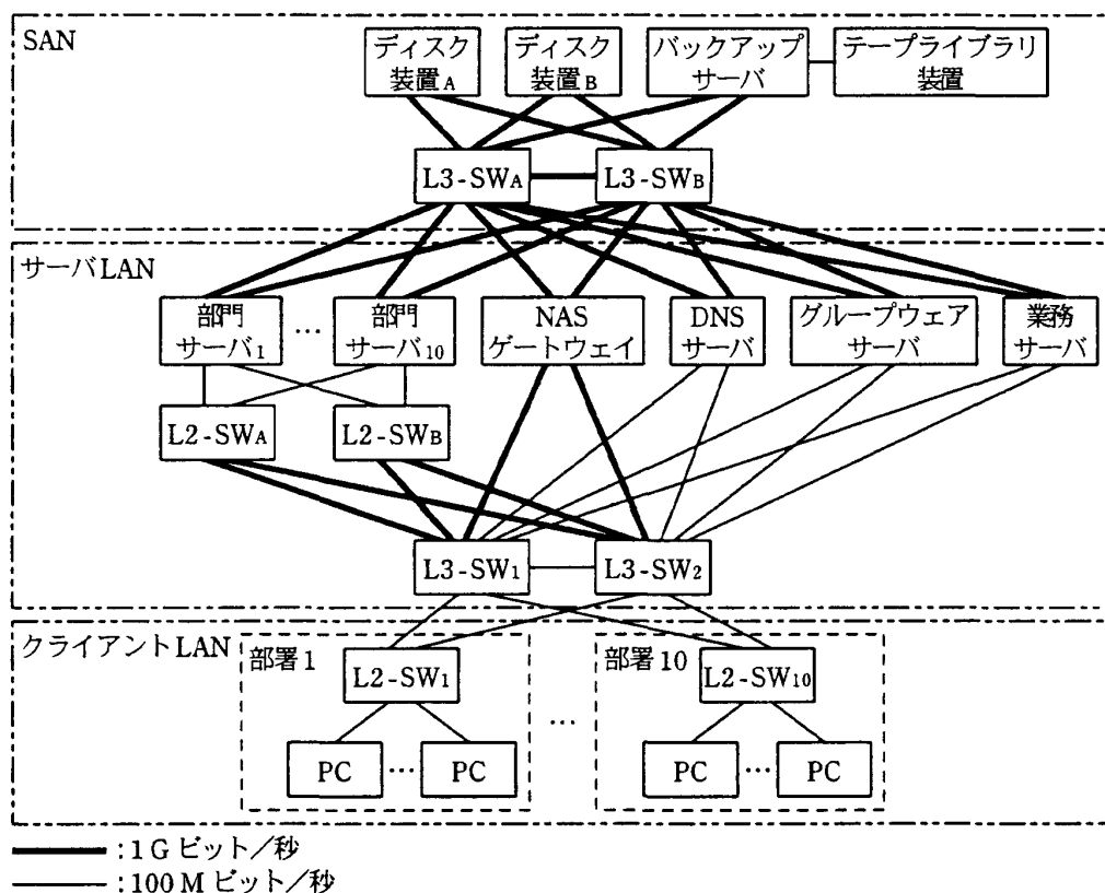
図 3 新社内システムの構成案（抜粋）
