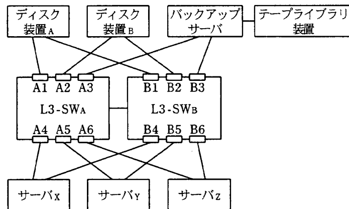
図 2 SAN の構成（概念）
