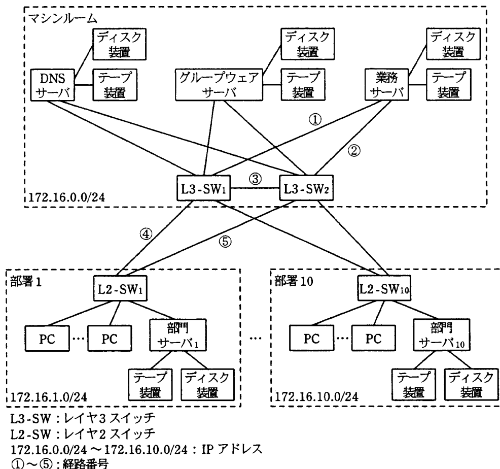
図1 社内システム構成（抜粋）
