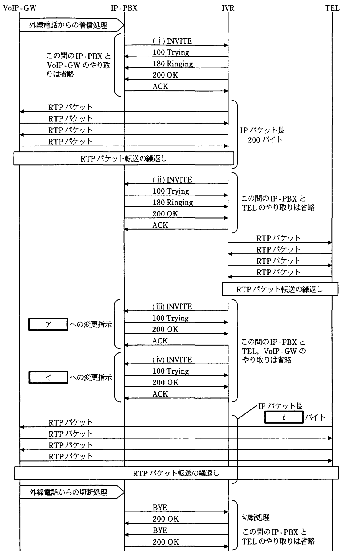
図3 動作シーケンス
