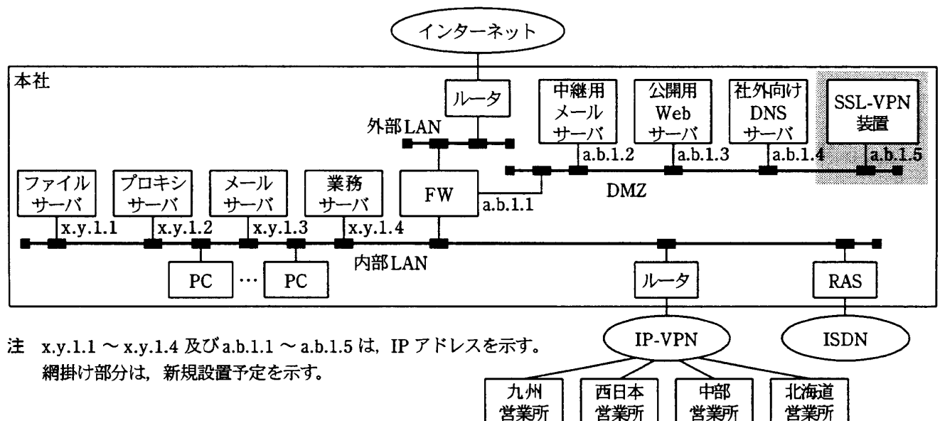
図1 Y社ネットワークの構成
