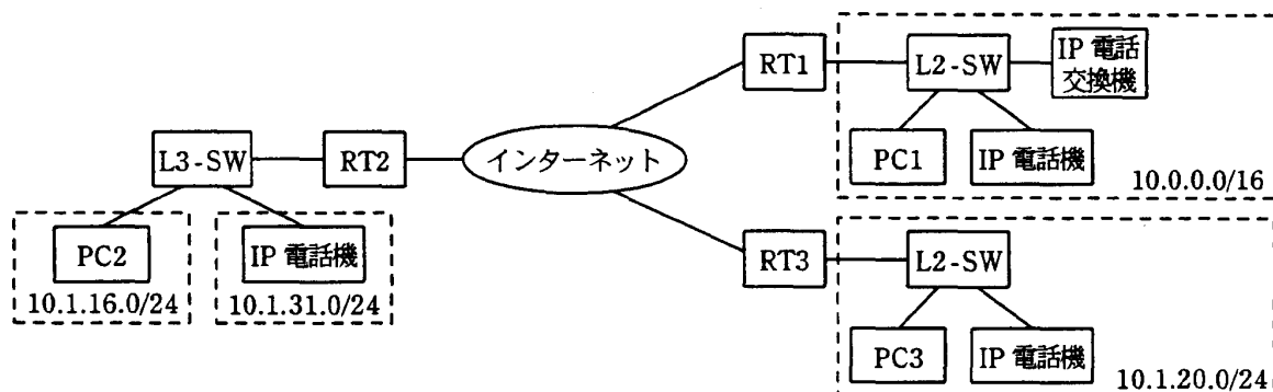
図 2 試験用ネットワークの構成
