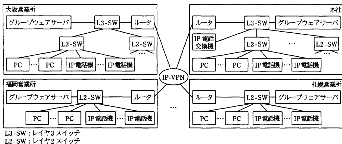
図1 現在のX社のネットワーク構成
