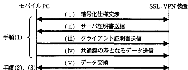
図 2 SSL 通信のシーケンス (概略)
