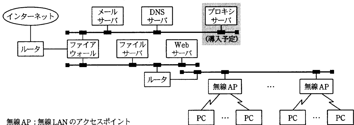
図1 A社ネットワークシステムの構成
