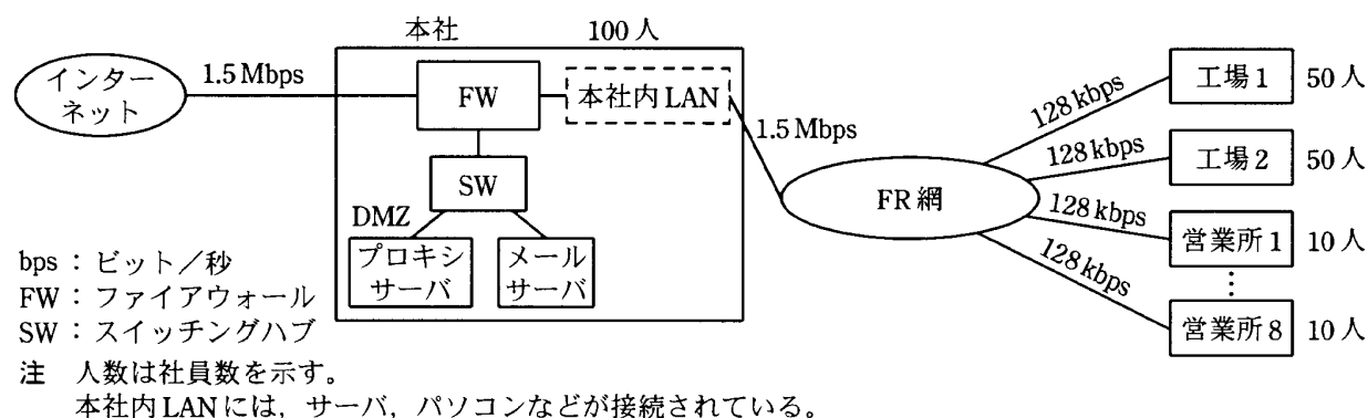
図1 S社の現行ネットワーク
