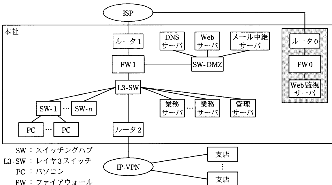
図1 A社のネットワーク構成
