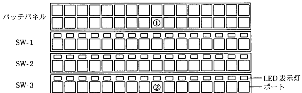
図 2 SW のラック搭載図
