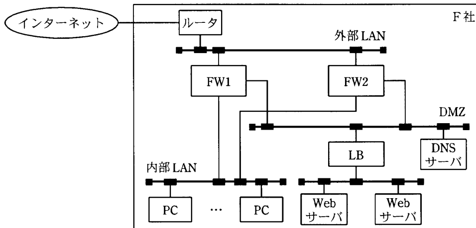
図 2 LB を使ったシステム構成
