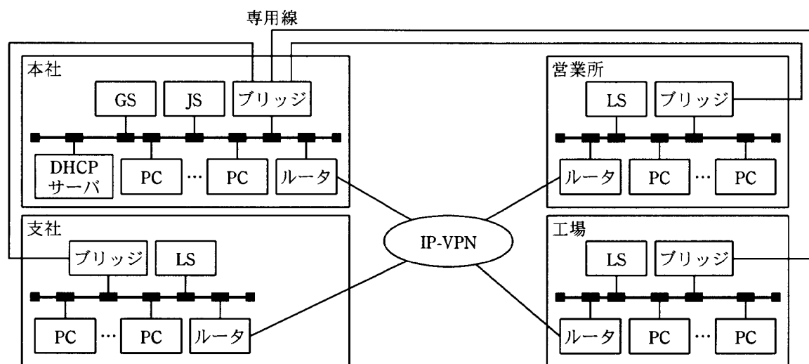
図 R社の移行期間のネットワーク構成
