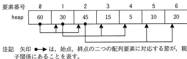
図2 図1のヒープの例に対応した配列 heap の内容
