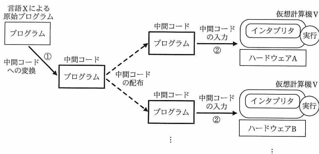
図 1 仮想計算機によるインタプリタ方式の実行例
