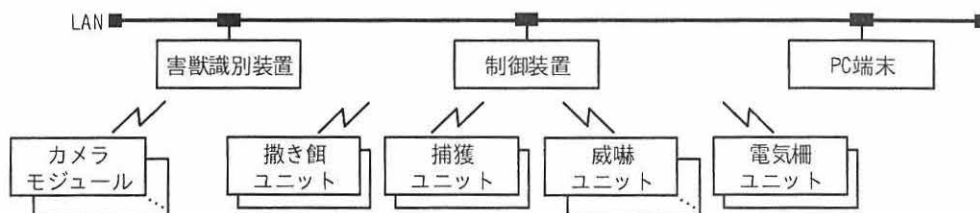
図2 監視システムの主な構成
