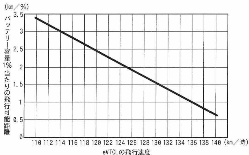
図 5 無風時における eVTOL の燃費と飛行速度の関係
