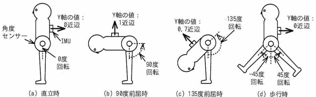
図 3 横から見た姿勢と角度センサー及び背中にある IMU の値との関係
