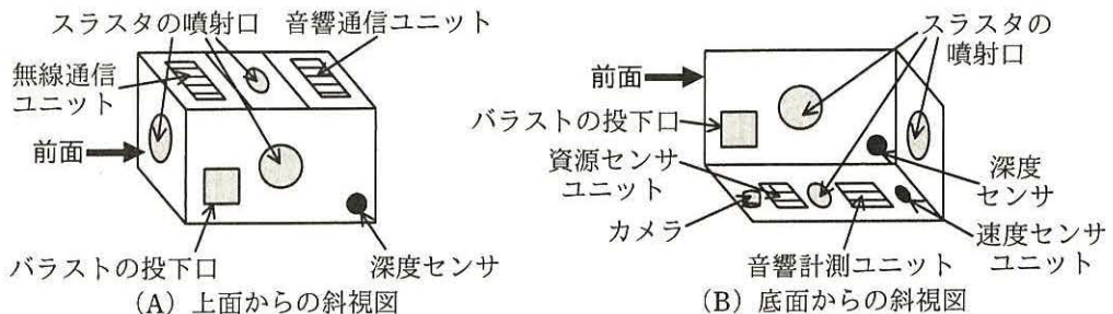
図2 探査機の外観
