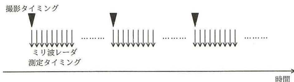
図10 ステレオカメラの撮影タイミングとミリ波レーダの測定タイミング
