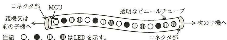
図 2 子機の外観
