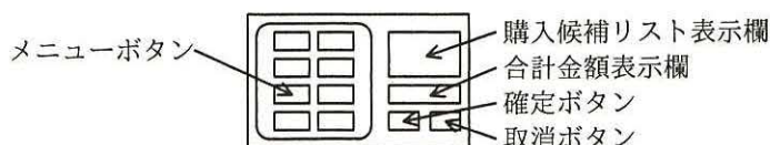
図3 注文中画面
