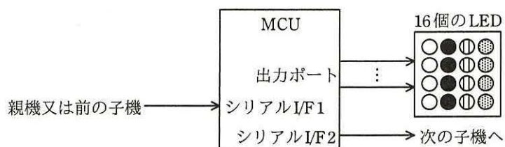
図 3 子機の構成
