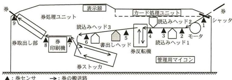
図1 改札機用乗車券処理装置の構成
