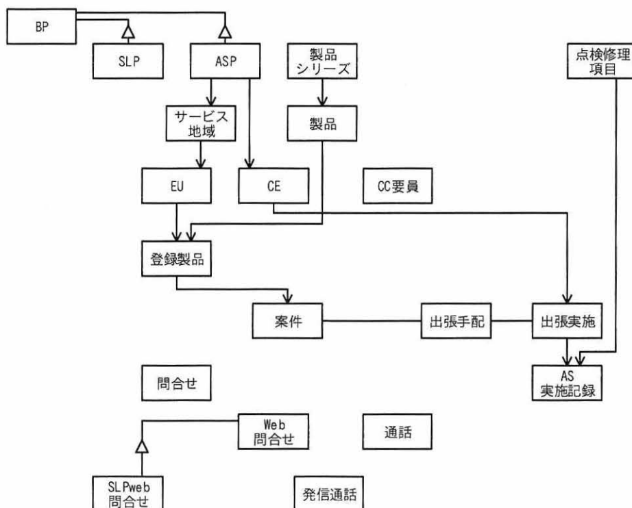
図1 現状の概念データモデル（未完成）
