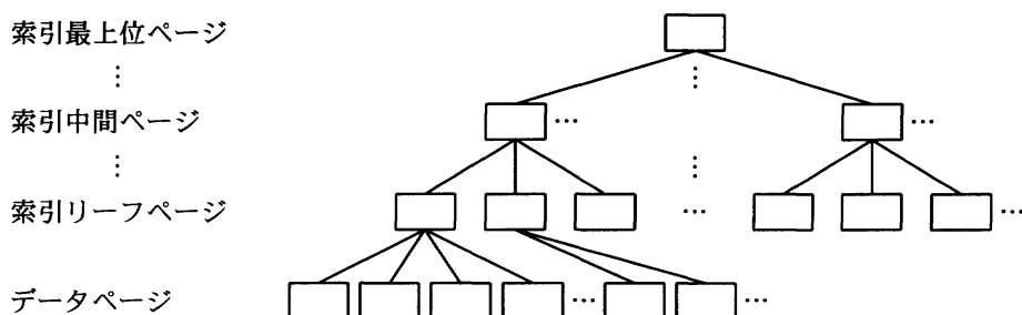
図1 索引とデータの物理構造
