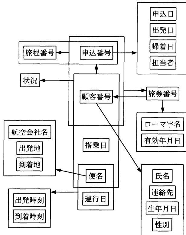
図2 航空券販売の主な関数従属性
