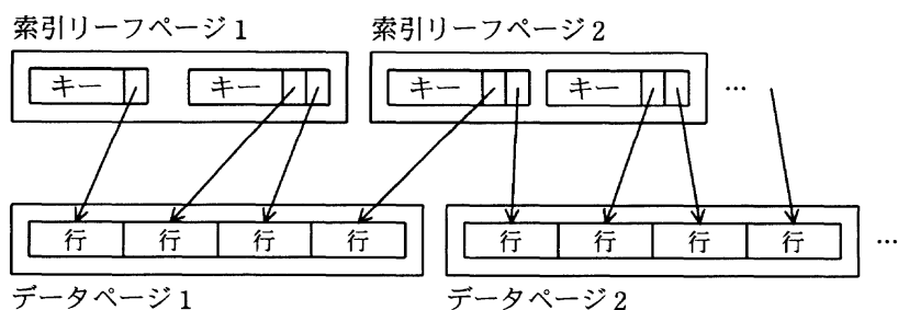
図 2 非ユニーク索引かつクラスタ索引
