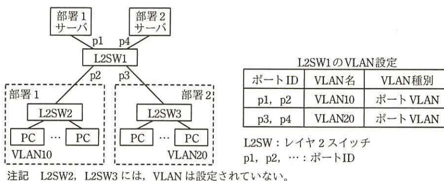
図 1 本社 LAN の構成 (抜粋)
