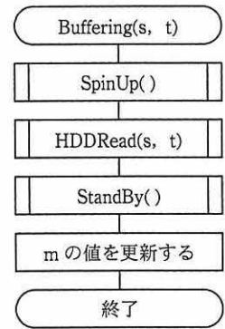
図5 サブルーチン Buffering(s, t)の流れ図
