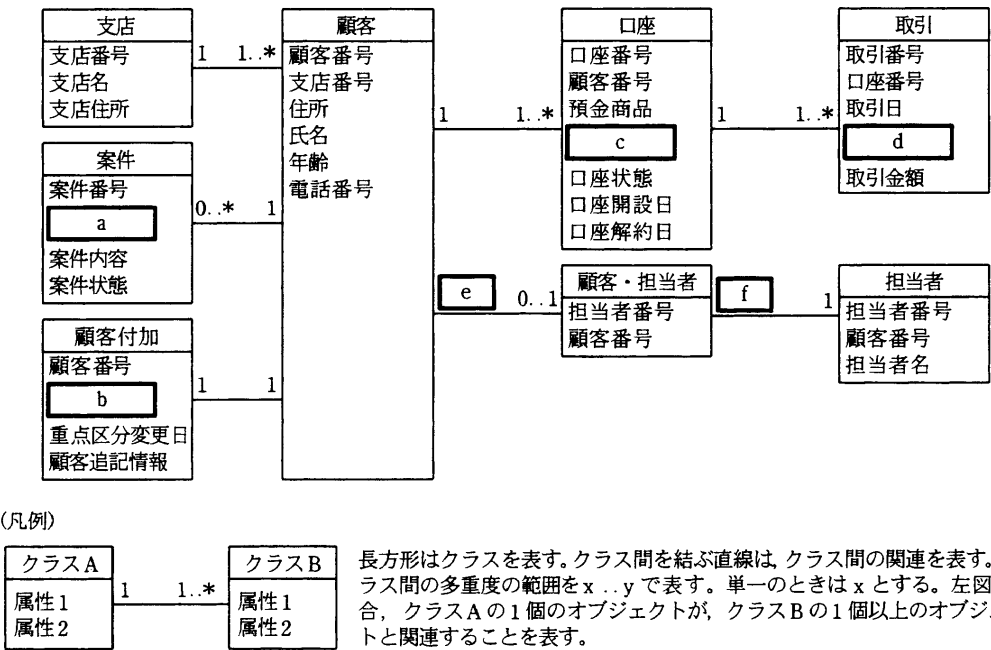
図 1 顧客管理支援システムのクラス図
